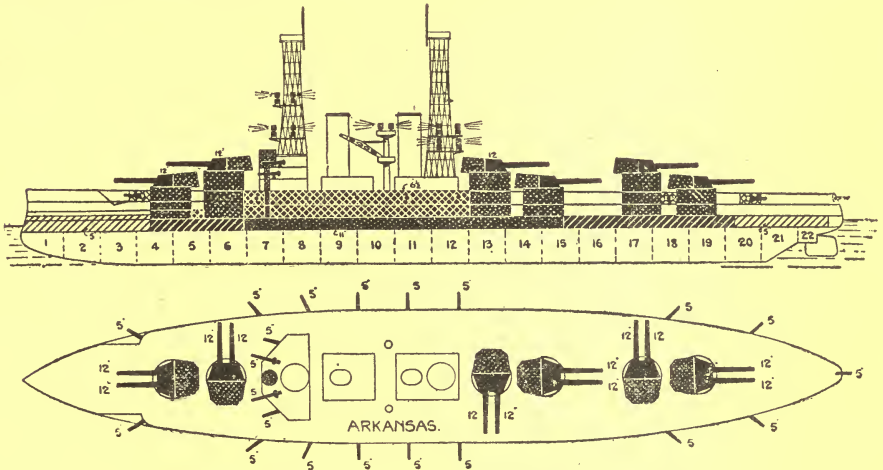
U. S. S. ARKANSAS
